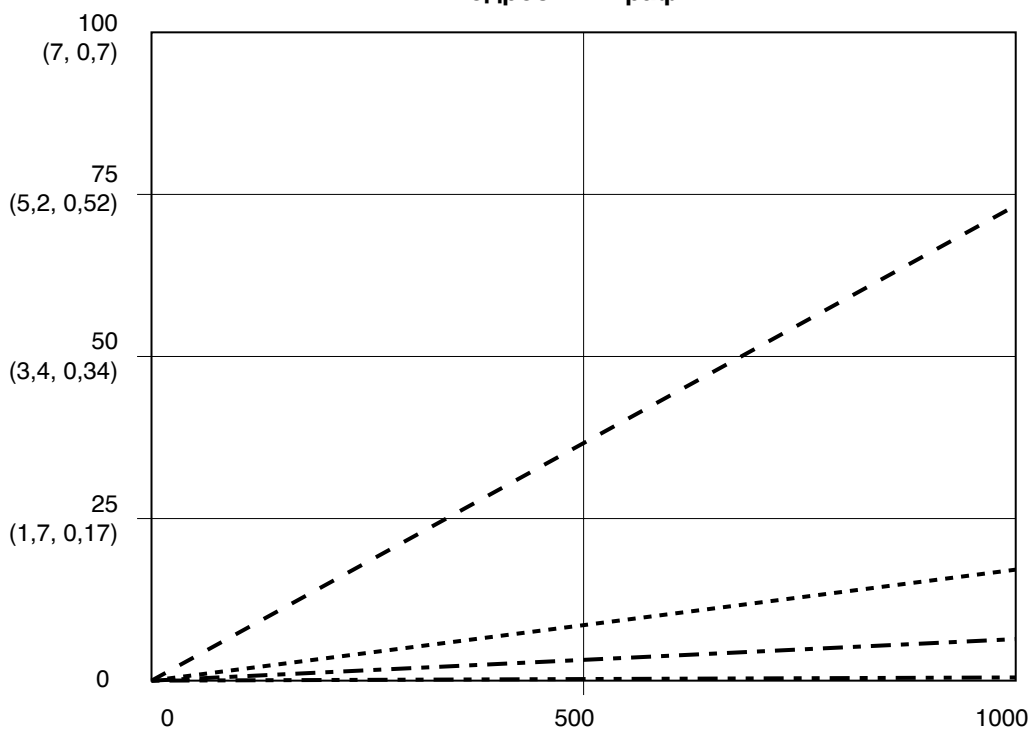
Рис. 59. Эксплуатационные характеристики при динамическом дозировании (соотношение = 20:1, вязкость жидкости = 90 спз, давление в контуре А = 0,7 МПа)
