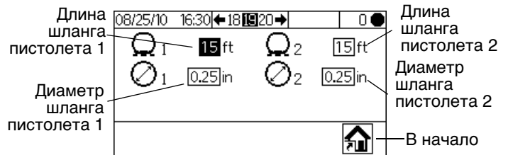
Рис. 38. Экран 19 (Настройка 2)
