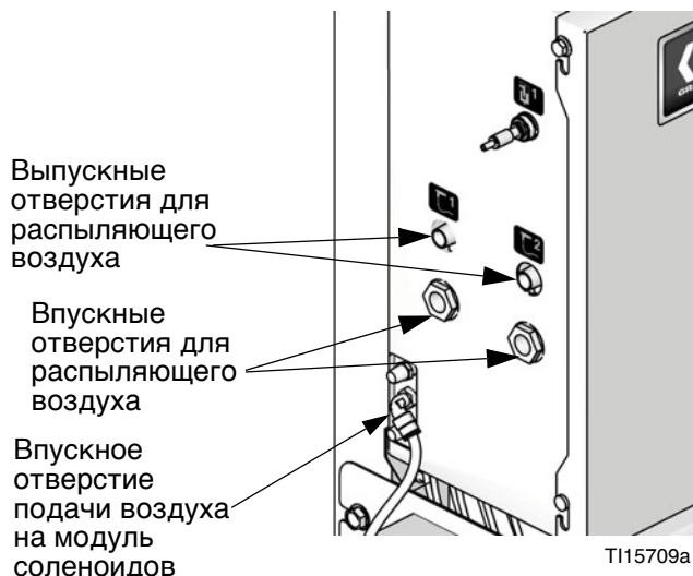
Рис. 4. Подсоединение линии подачи распыляющего воздуха
