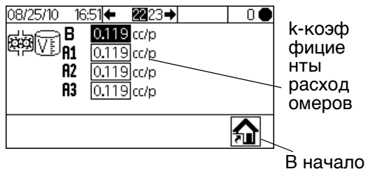
Рис. 44. Экран 22 (Калибровка 1)
