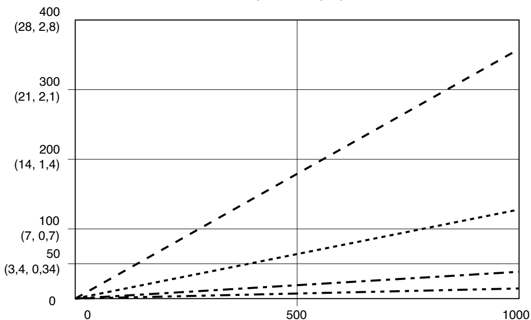
Рис. 57. Эксплуатационные характеристики при динамическом дозировании (соотношение = 5:1, вязкость жидкости = 90 спз, давление в контуре А = 0,7 МПа)
