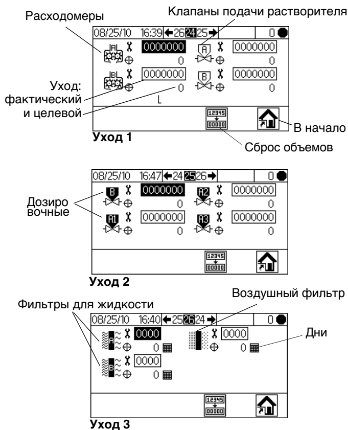
Рис. 43. Экраны 24–26 (Уход 1–3)
