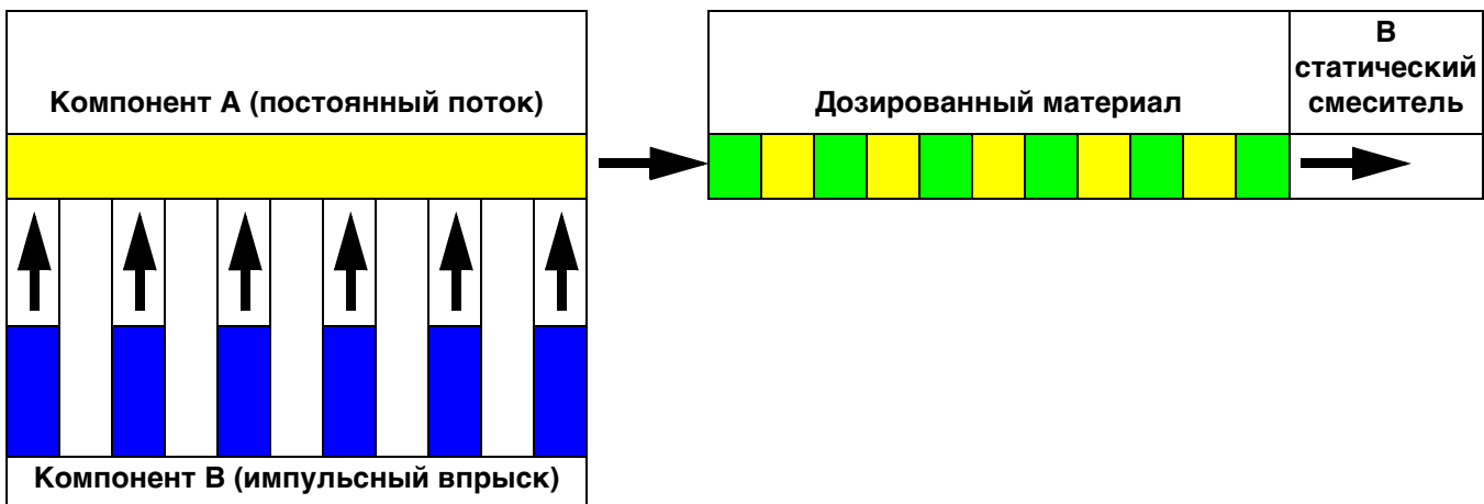
Рис. 53. Схема работы при динамическом дозировании
