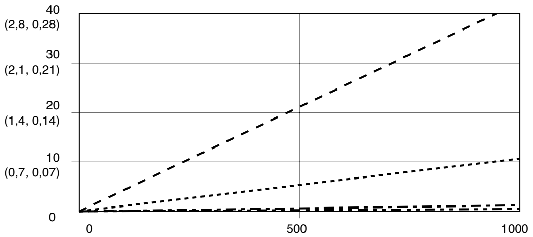
Рис. 60. Эксплуатационные характеристики при динамическом дозировании (соотношение = 30:1, вязкость жидкости = 90 спз, давление в контуре А = 0,7 МПа)
