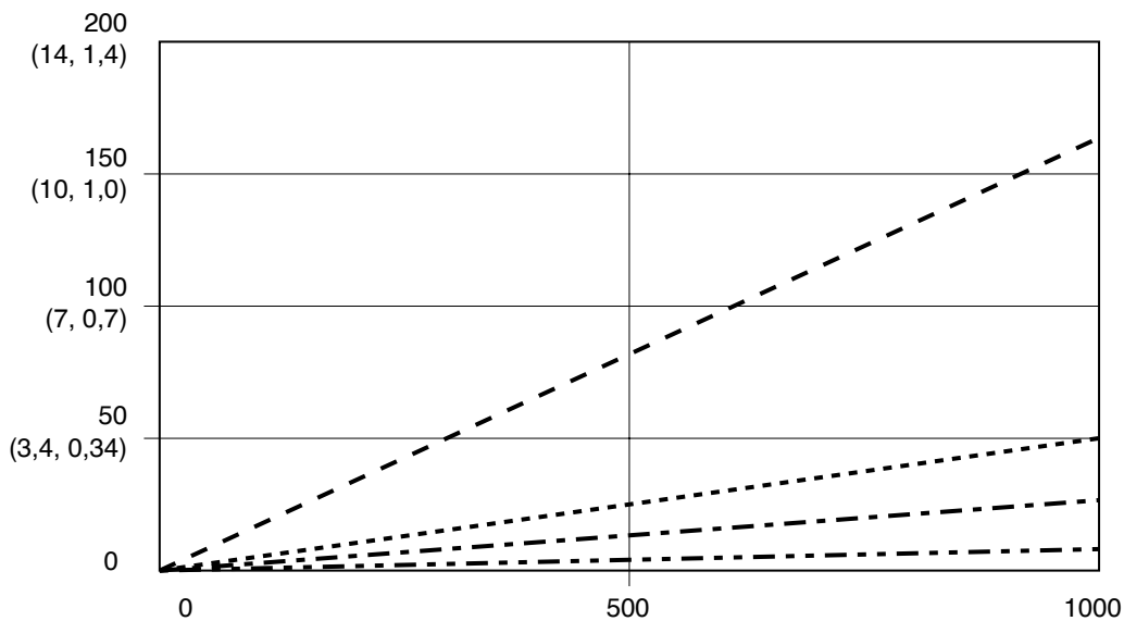
Рис. 58. Эксплуатационные характеристики при динамическом дозировании (соотношение = 10:1, вязкость жидкости = 90 спз, давление в контуре А = 0,7 МПа)
