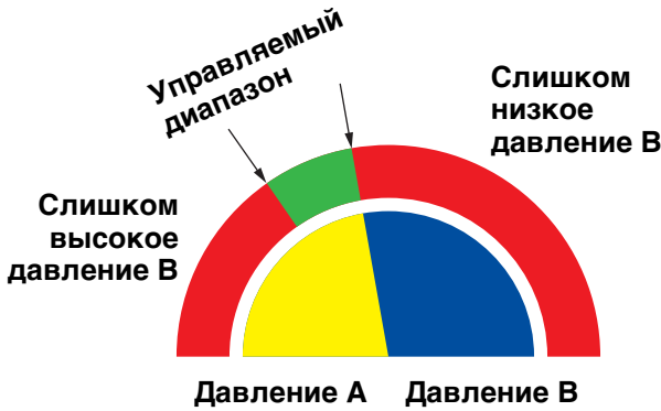
Рис. 51. Управляемый диапазон давления А и В при выборе ограничителя правильного размера
