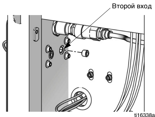
Рис. 5. Вход для рециркуляции краски
