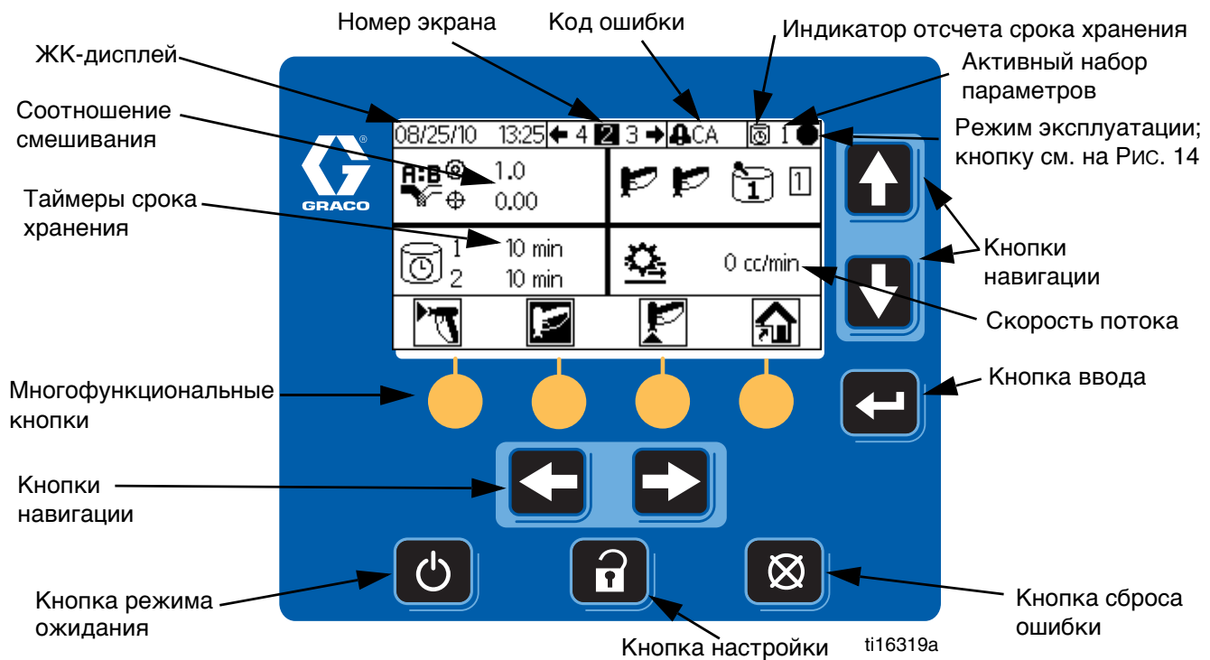
Рис. 13. Модуль дисплея
