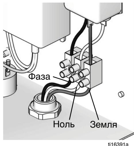
Рис. 9. Электрическое соединение блока управления
