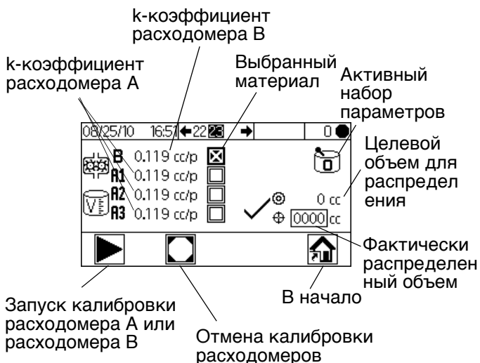
Рис. 45. Экран 23 (Калибровка 2)
